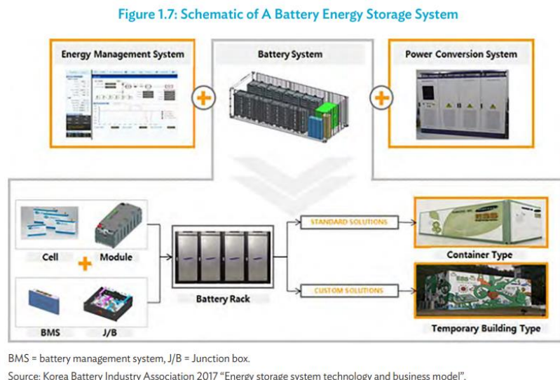
Figura 2 – Componenti di un BESS
